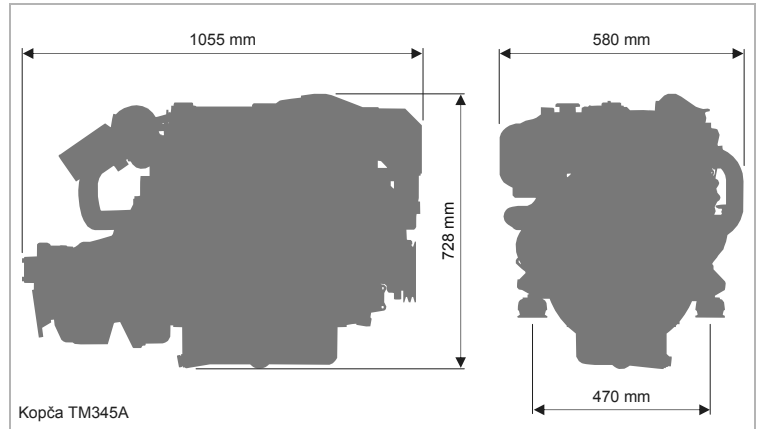
Kopča TM345A
